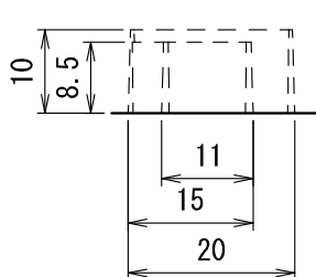
側面ロックアウトA 詳細 (1/1)
