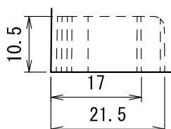
側面ロックアウトC 詳細 (1/1)
