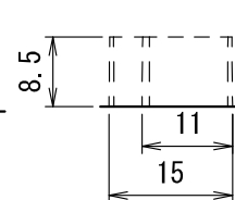
側面ロックアウトB 詳細 (1/1)
